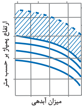
نمودار ۱: منحنی آبدهی-فشار (Q-H)
