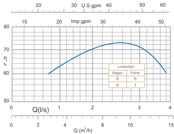
منحنی راندمان / Efficiency Curve
