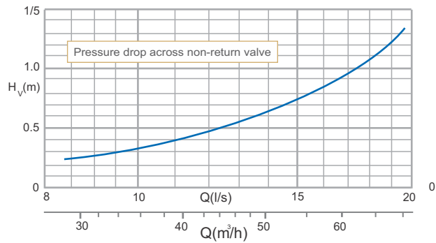
Valve Losses Curve / منحنی افت سوپاپ ۴ اینچ
