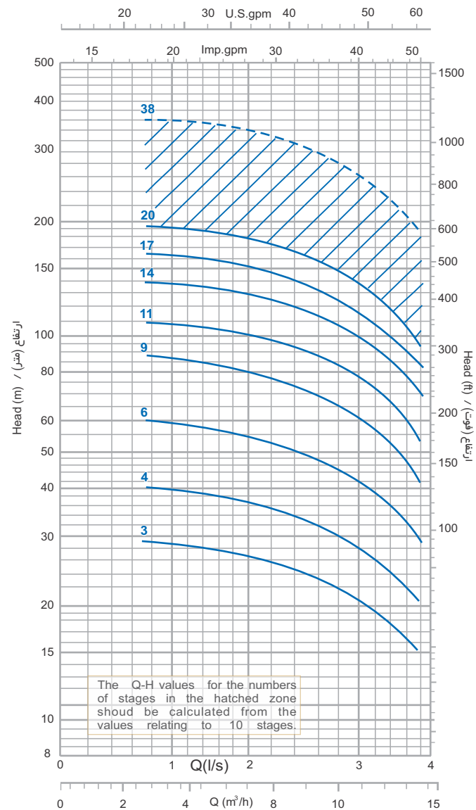
منحنی آبدهی-فشار / Q-H Curve
