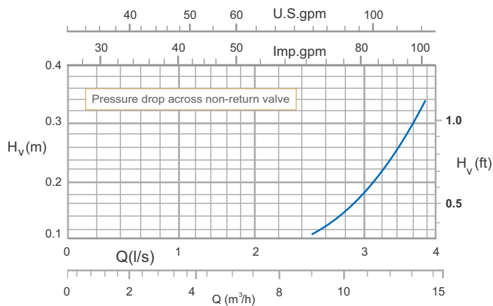
منحنی افت سوپاپ ۱/۵ اینچ / Valve Losses Curve
