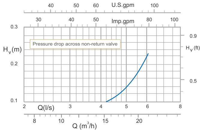
منحنی افت سوپاپ ۲ اینچ / Valve Losses Curve
