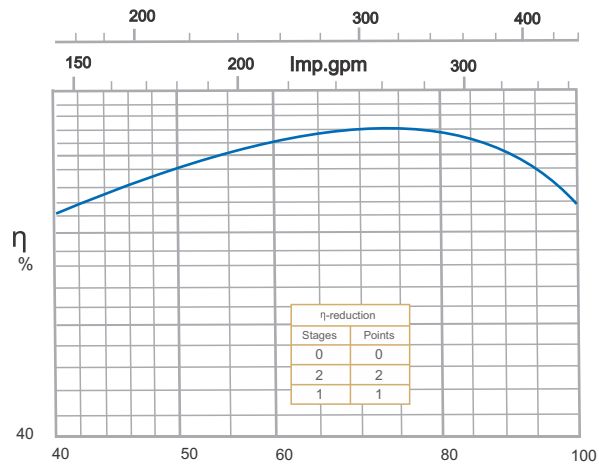
Efficiency Curve / منحنی راندمان
